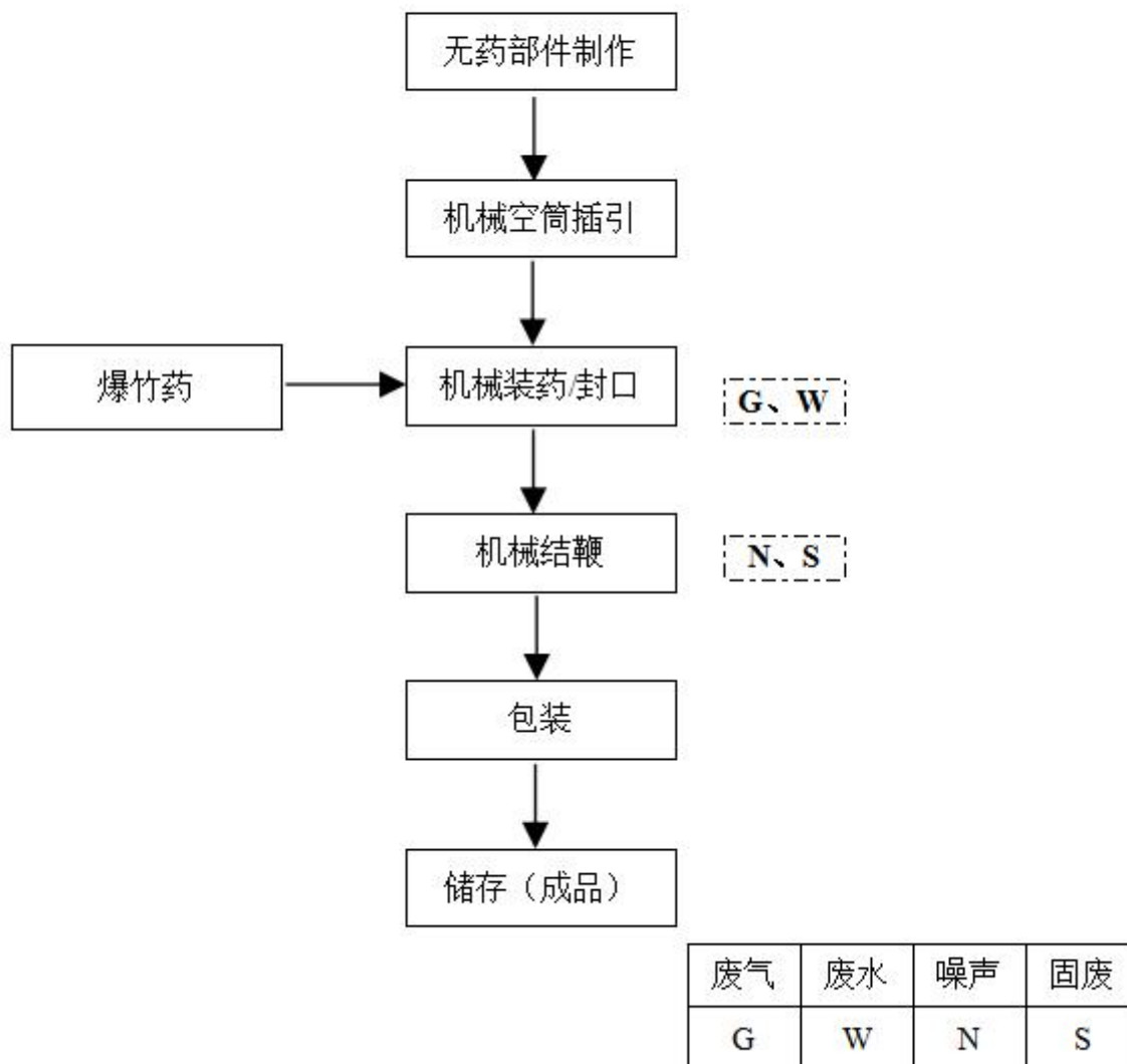
图1 鞭炮生产工艺流程及产污节点图
