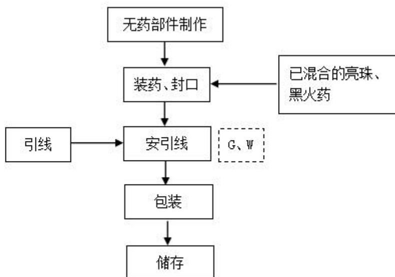
图2 喷花类产品生产工艺流程及产污节点图
