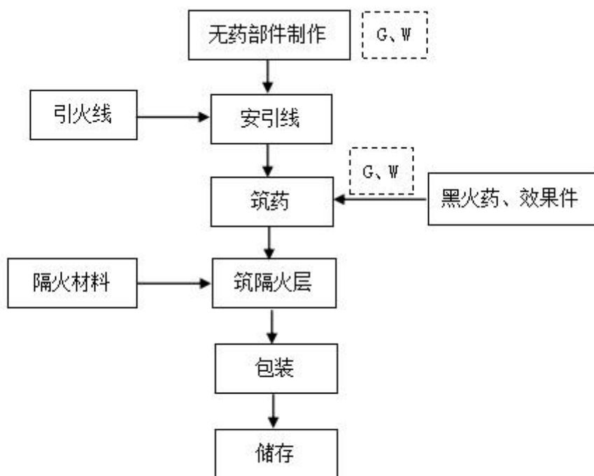
图3 吐珠类产品生产工艺流程及产污节点图
